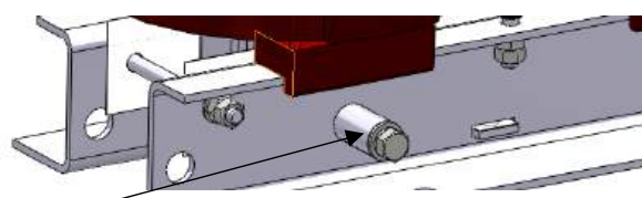
Рис. 33. Порядок монтажа выкатного элемента с трансформатором собственных нужд в отсек кабельных присоединений
