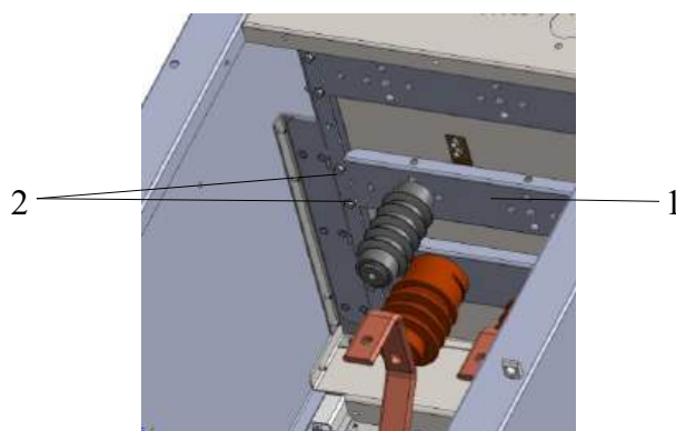
Рис. 38. Планка с ОПН
