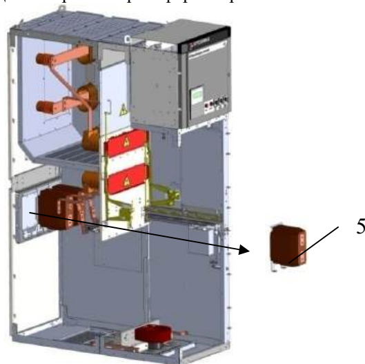
Рис. 39. Порядок демонтажа измерительных трансформаторов тока
