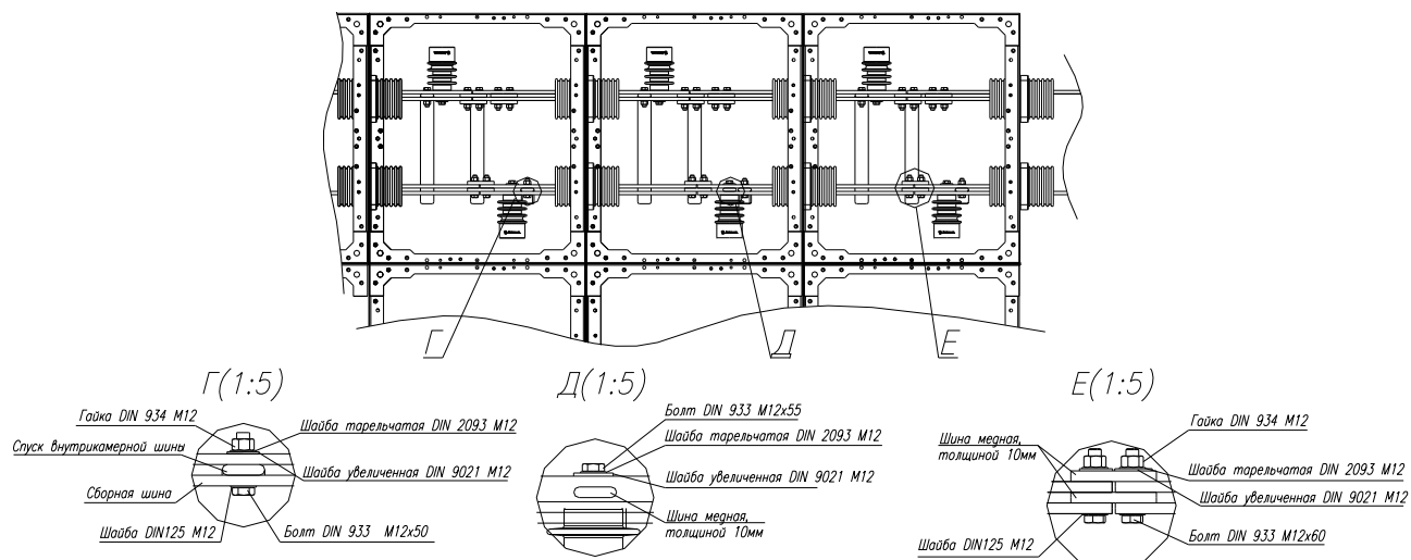
Рис. 28. Монтаж сборных шин 2500 А (вид сверху на шкафы КРУ)
