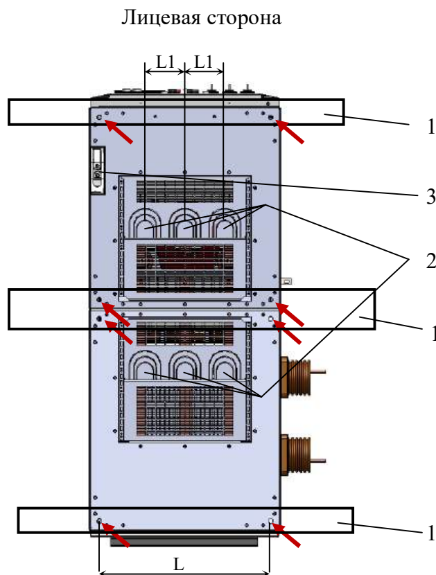
Рис. 20. Установочные размеры шкафов КРУ, размещение закладных швеллеров и отверстий для прохода силовых и контрольных кабелей. Вид сверху на дно шкафа КРУ
