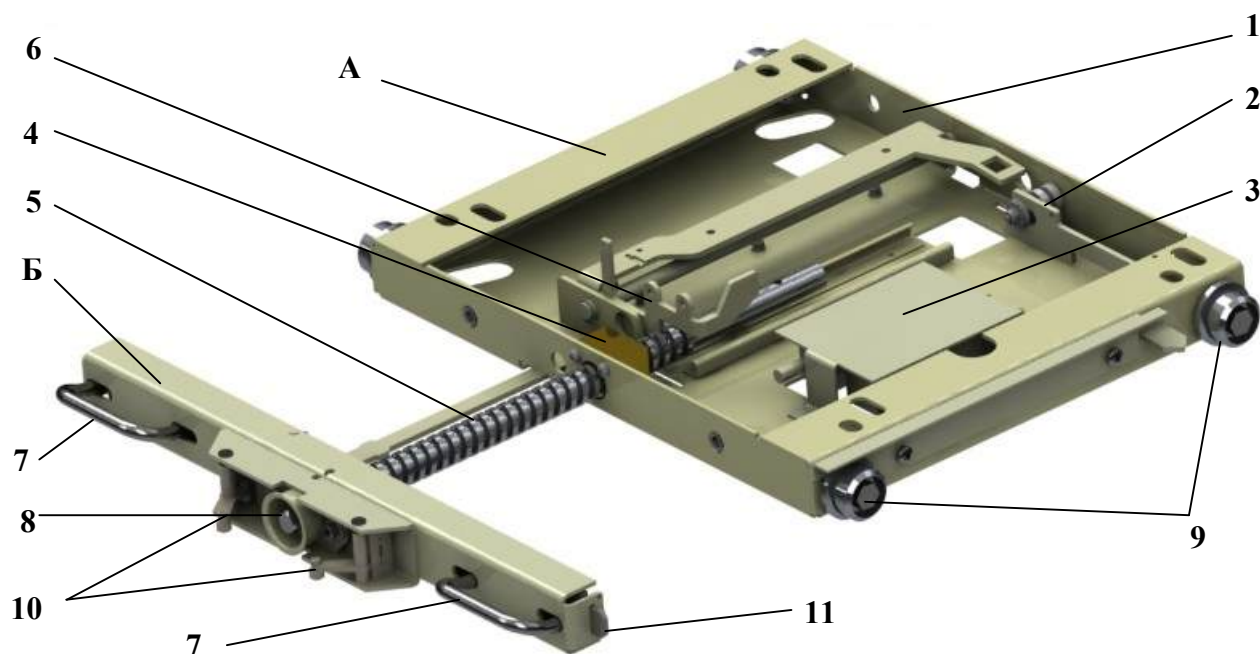
Рис. 8. Тележка аппаратная:
