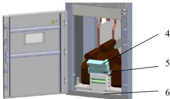
Рис. 32а. Порядок монтажа выкатного элемента с измерительными трансформаторами напряжения в отсек кабельных соединений
