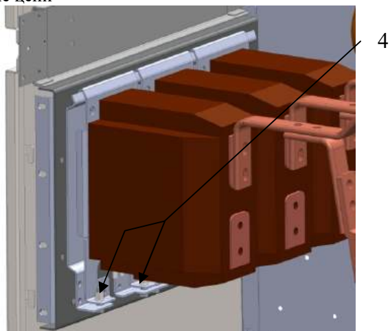
Рис. 39. Порядок демонтажа измерительных трансформаторов тока
