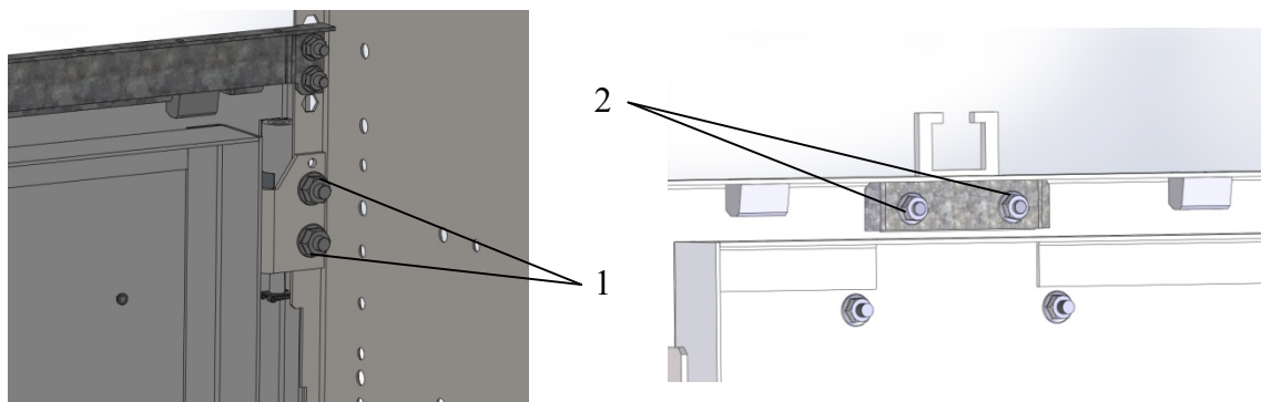
Рис. 206. Крепление петель дверей и деблокирующей планки (вид изнутри)
