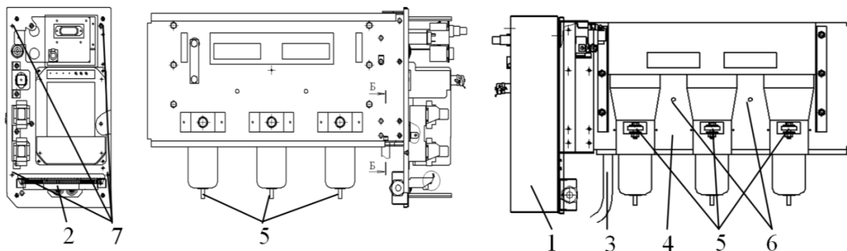
Рис. 23. Крепление силового выключателя (на примере ВВ/ТЕЛ):
