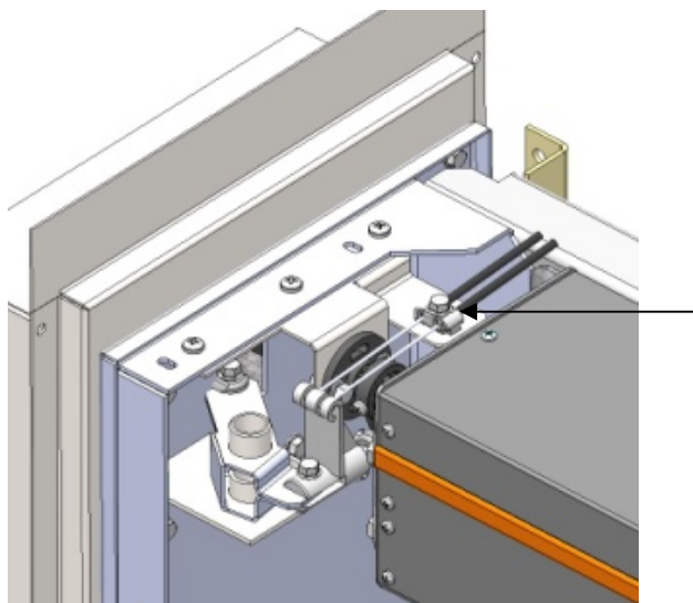
Рис. 5.1 Установка тросика в выключателе VM12
