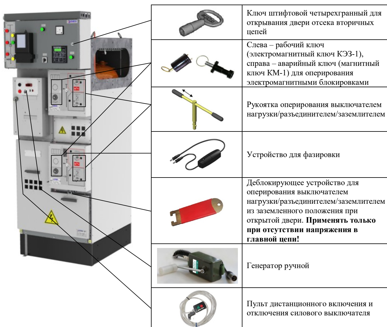
Рис. 5. Принадлежности КСО
