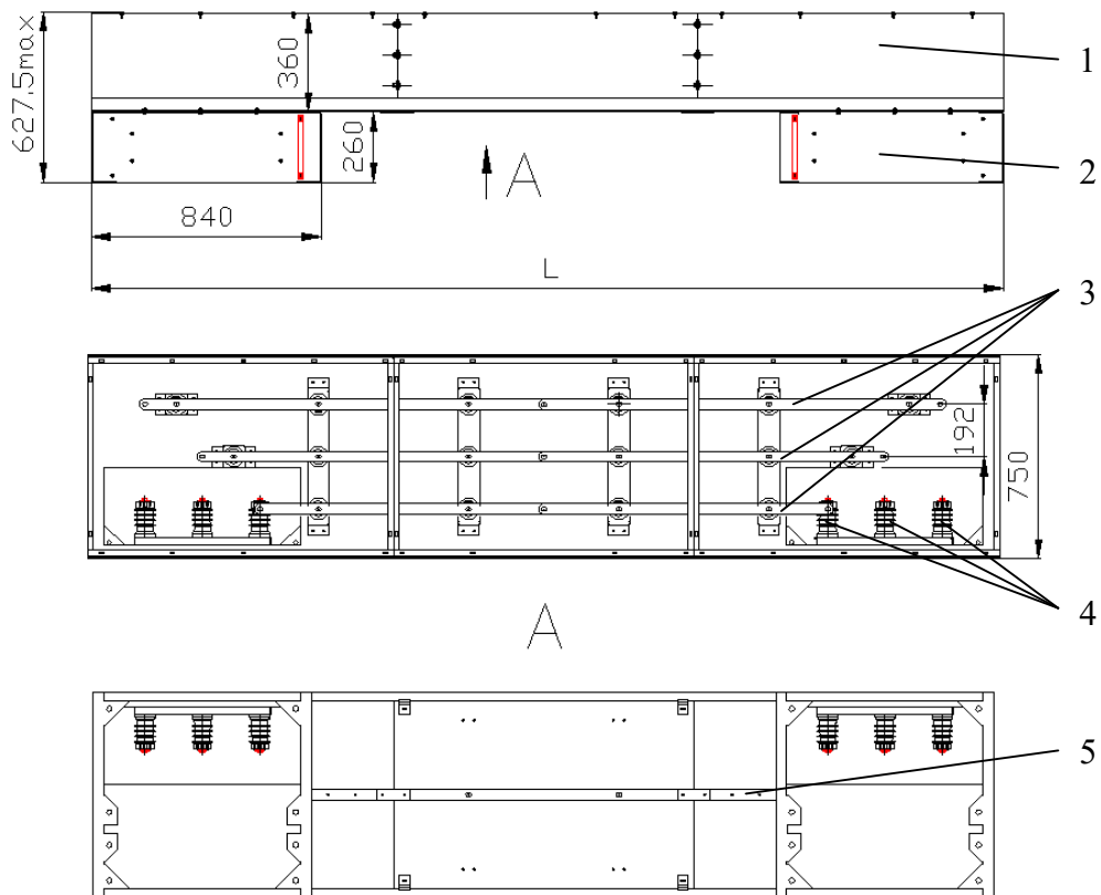
Рис. 4. Шинный мост:
