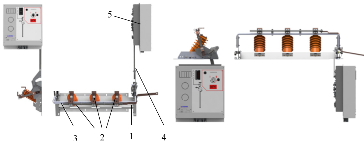
Рис. 8. Заземлитель SL
